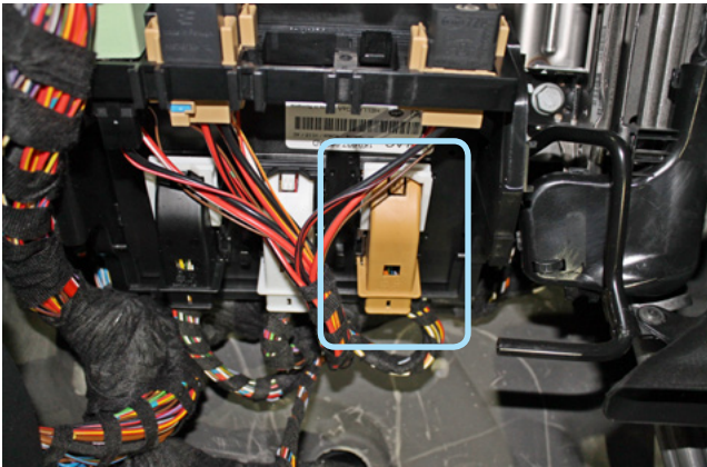
Фото 3.15. Местоположение коричневого разъёма на блоке BCM
