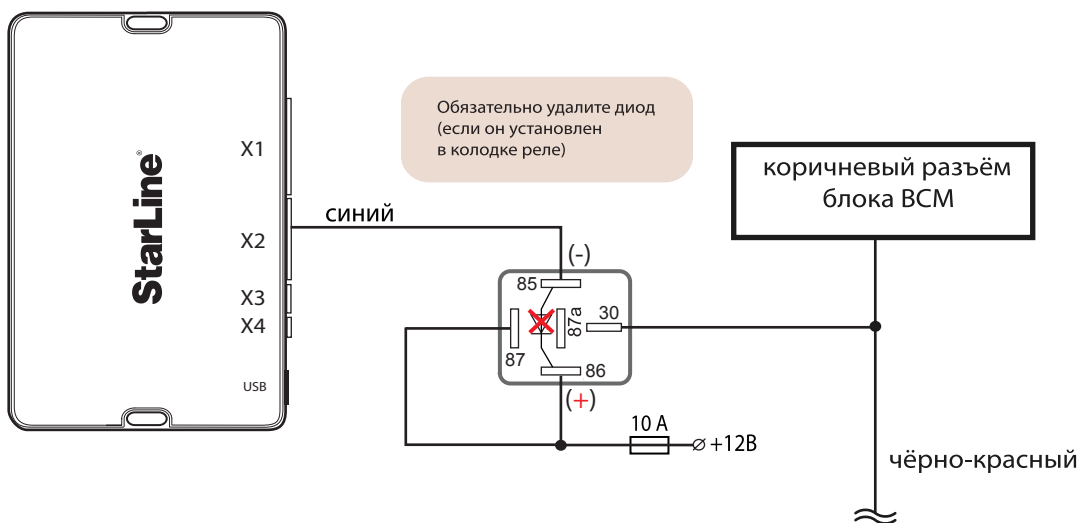
Схема 1. Имитация нажатия педали тормоза
