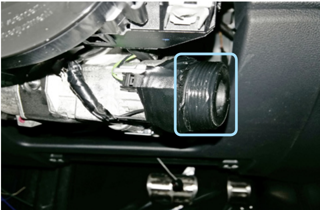
Фото 3.15. Расположение антенны BP-03 на замке зажигания
