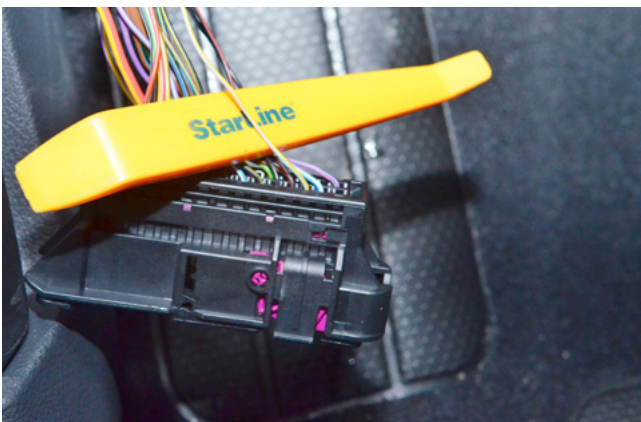
Фото 3.15. Управление замком багажника (жёлто-серый)
