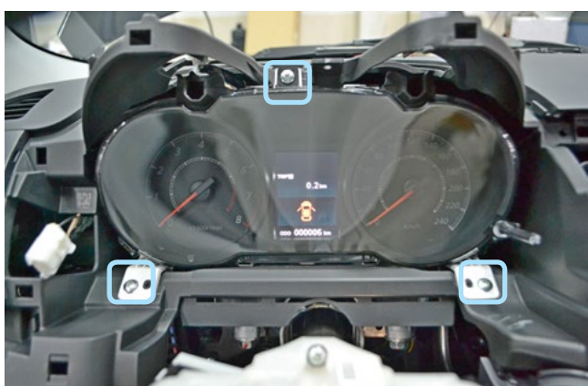
Фото 1.31. Саморезы крепления панели приборов
