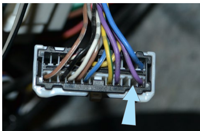
Фото 3.6. Управление центральным замком (закрытие - pin 19)
