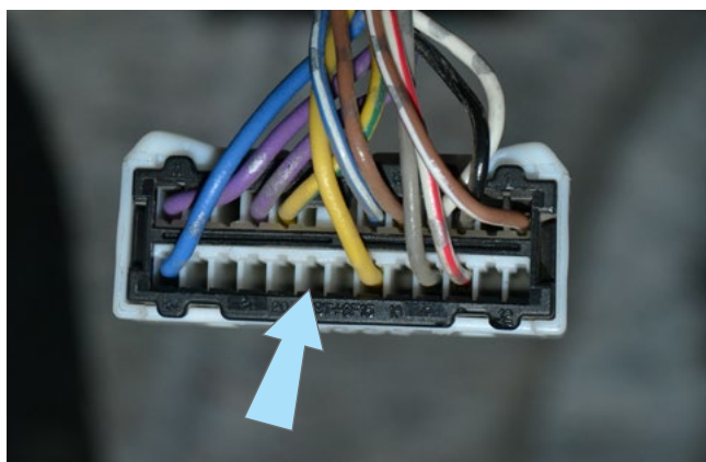
Фото 3.7. Управление центральным замком (открытие - pin 10)
