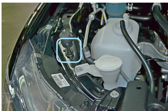
Фото 2.7. Возможное место установки концевика капота
