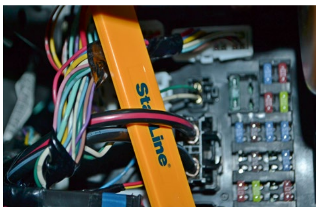
Фото 3.13. Питание +12В (чёрно-красный)
