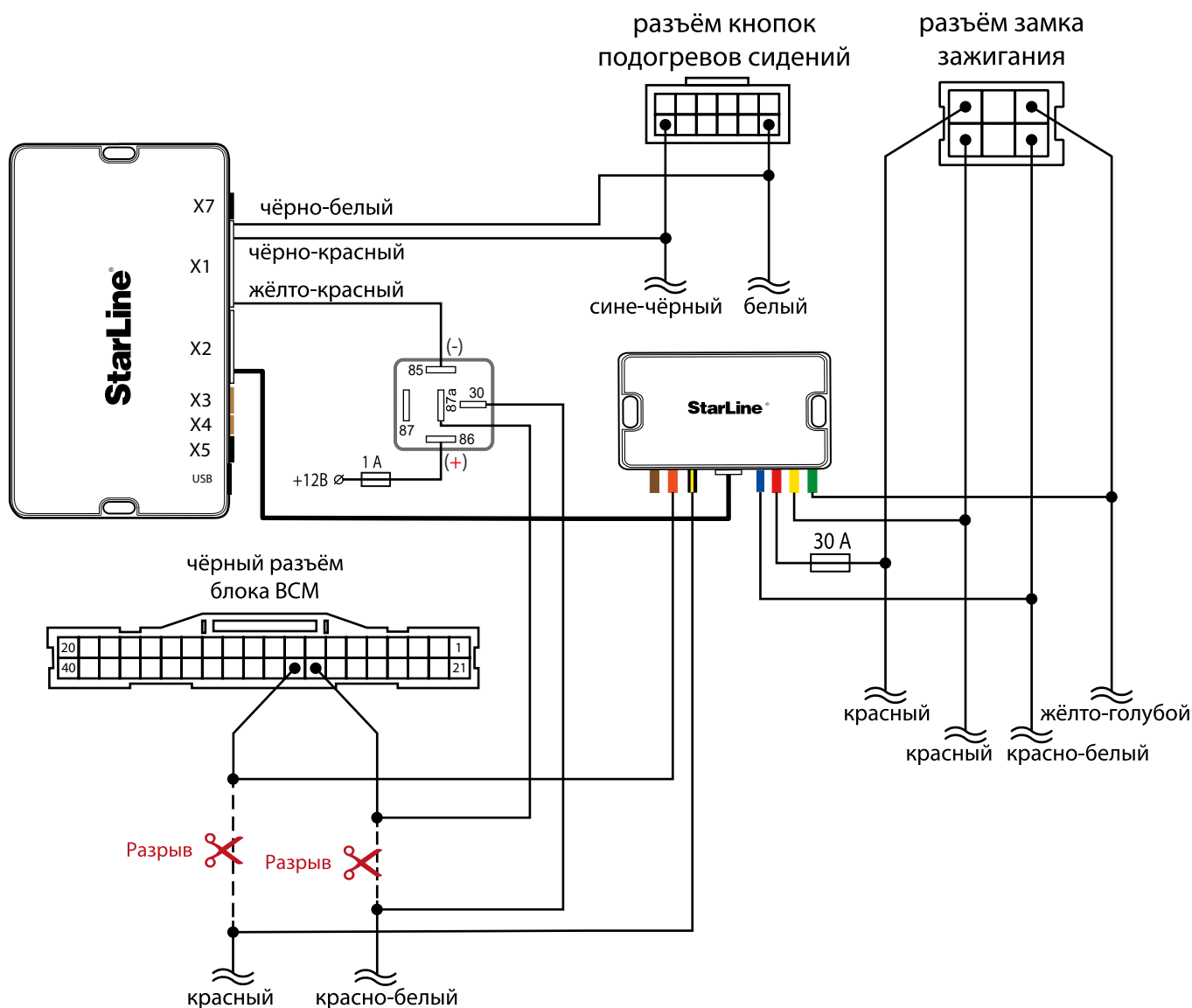
Схема 1. Подключение цепей автозапуска двигателя и управления подогревами сидений
