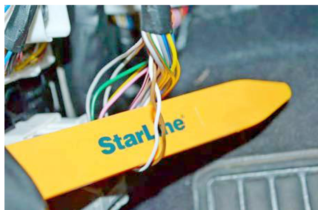
Фото 3.3. Шина CAN-A (коричневый и белый)
