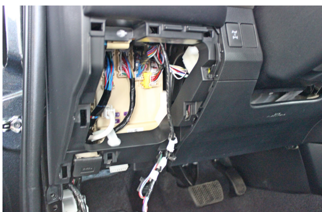
Фото 1.5. Декоративная накладка снята
