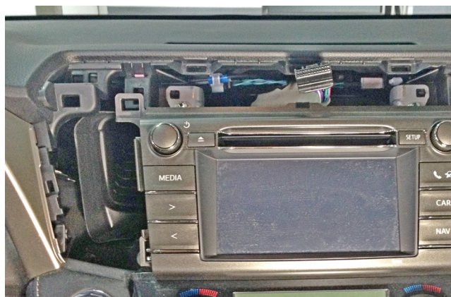
Фото 1.9. Воздуховод слева от магнитолы снят
