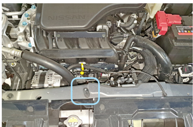
Фото 2.8. Возможное место установки концевика капота
