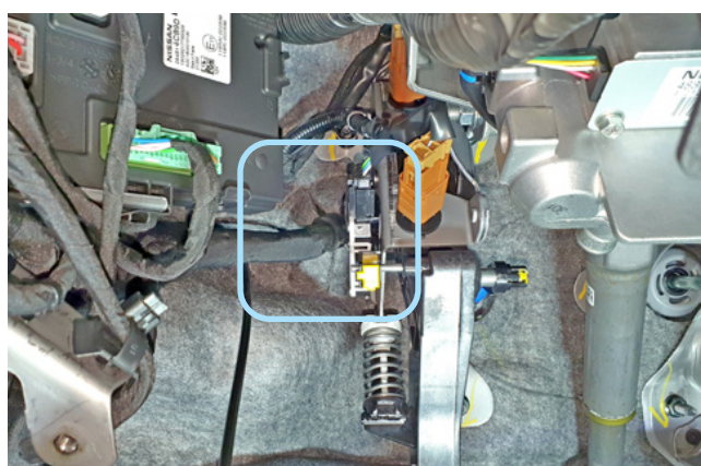
Фото 2.9. Штатный уплотнитель. Вид со стороны салона
