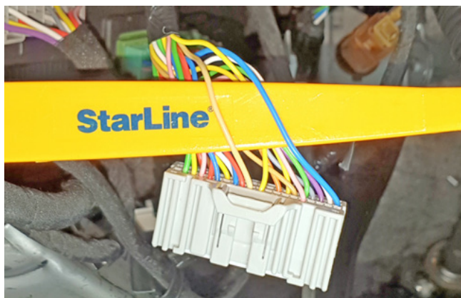
Фото 3.6. Управление центральным замком (бежевый и синий)
