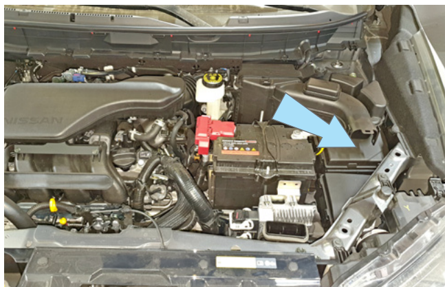
Фото 2.11. Возможное место установки подкапотного блока R6
