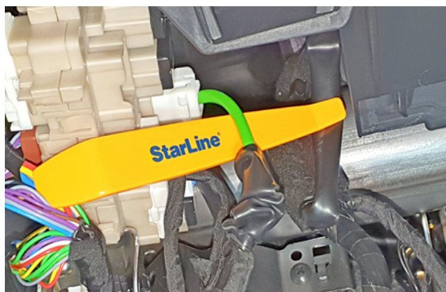
Фото 3.12. Питание +12В (зелёный)
