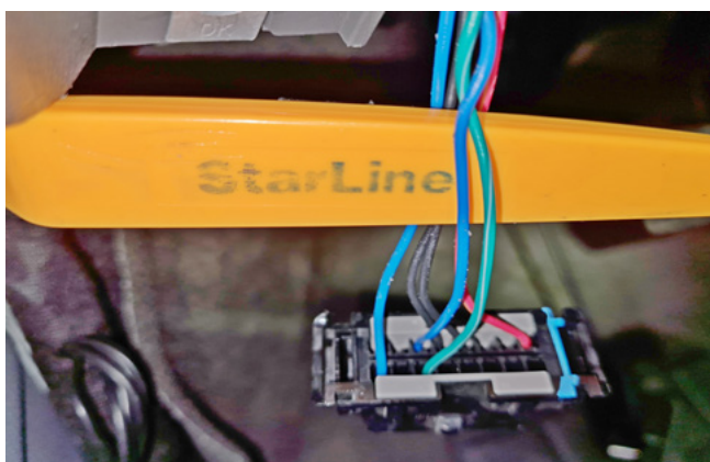
Фото 3.4. Шина CAN-B (синий и зелёно-серый)
