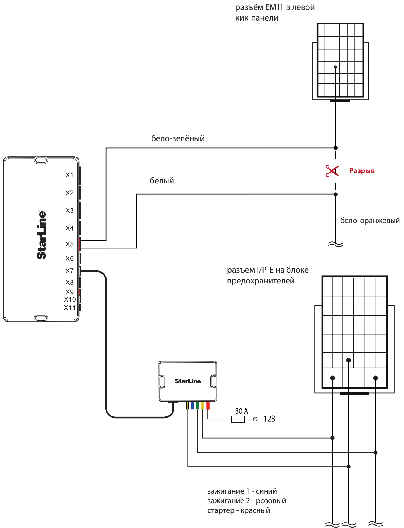
Схема 1. Подключение цепей автозапуска двигателя и обхода штатного иммобилайзера
