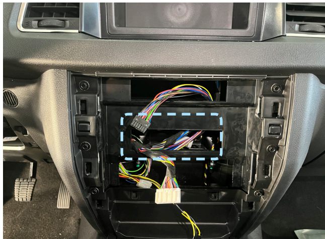
Фото 2.10. Пример расположения центрального блока охранно-телематического комплекса
