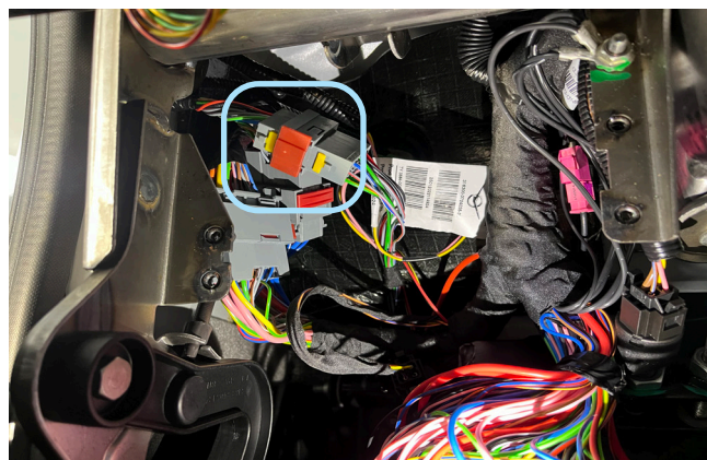
Фото 3.6. Местоположения разъёма выходящего из жгута двери водителя
