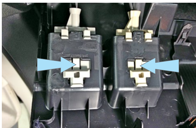
Фото 1.11. Фиксаторы крепления ручек отпирания капота и лючка бензобака
