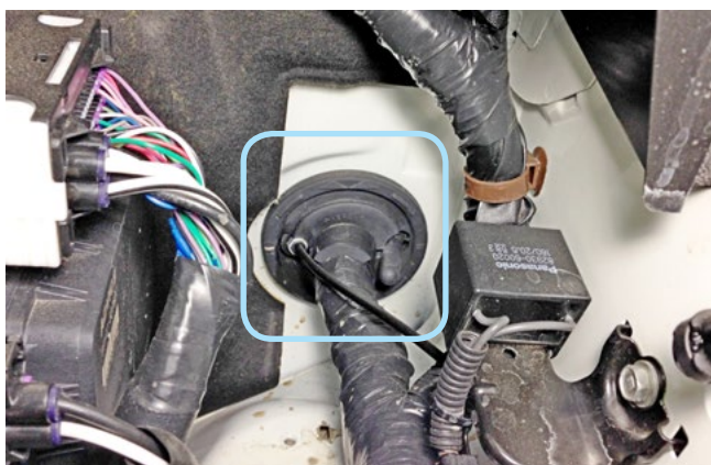
Фото 2.5. Штатный уплотнитель. Вид со стороны капота
