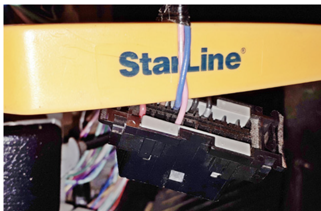
Фото 3.5. Шина CAN-B (синий и розовый)
