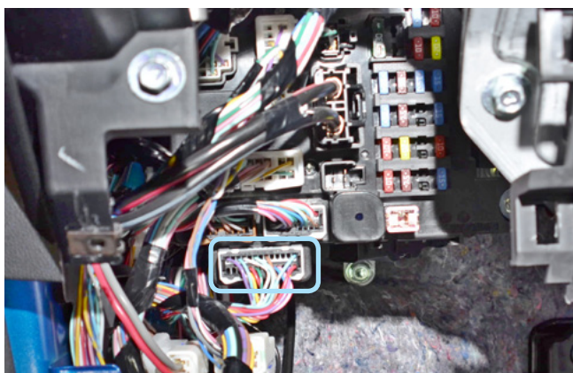
Фото 3.6. Местоположение разъёма C-411
