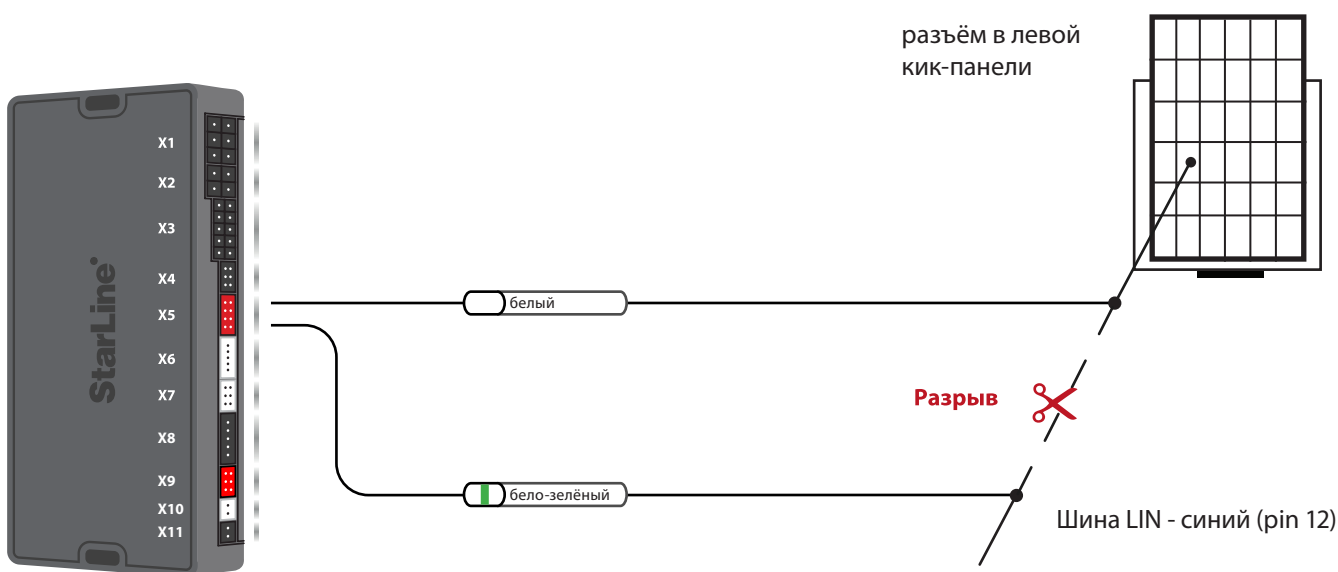
Схема 1. Подключение цепей обхода штатного иммобилайзера
