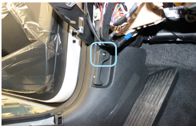
Фото 1.11. Винт крепления ручки отпирания капота
