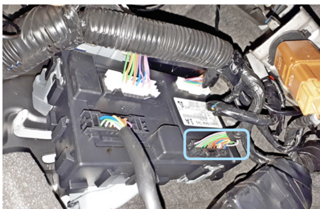
Фото 3.6. Местоположение разъёма M92
