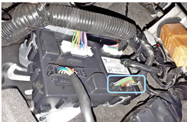
Фото 3.2. Местоположение разъёма M92
