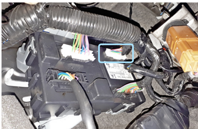
Фото 3.4. Местоположение разъёма M96
