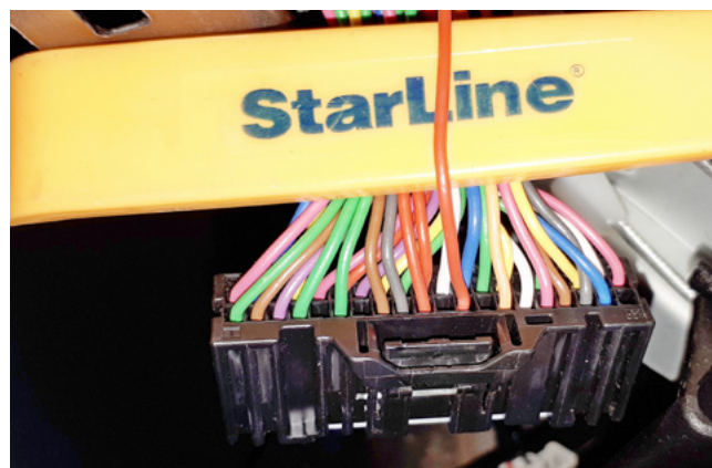
Фото 3.7. Имитация нажатия педали тормоза (красный)
