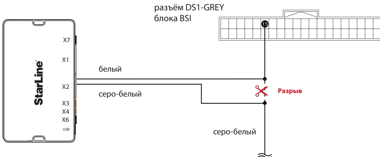
Схема 1. Подключение LIN-шины
