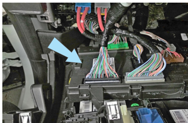
Фото 1.6. Блок BSI снят
