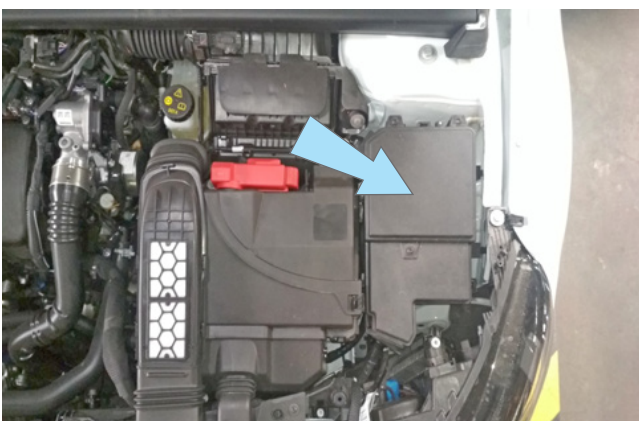
Фото 2.8. Возможное место установки подкапотного блока R6
