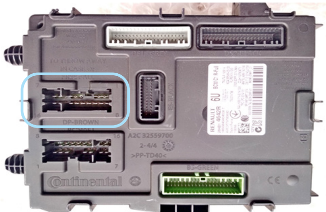
Фото 3.1. Местоположение разъёма на блоке BSI
