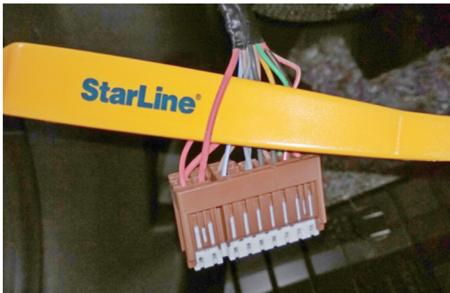
Фото 3.10. Питание +12В (красный)
