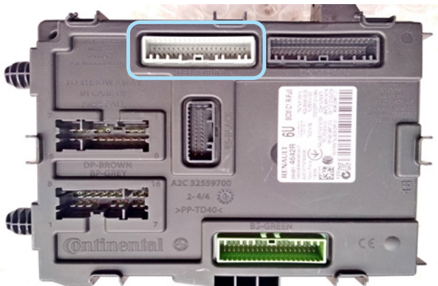
Фото 3.5. Местоположение разъёма на блоке BSI
