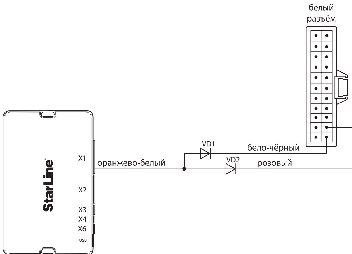
Схема 2. Подключение сенсорных датчиков ручек передних дверей
