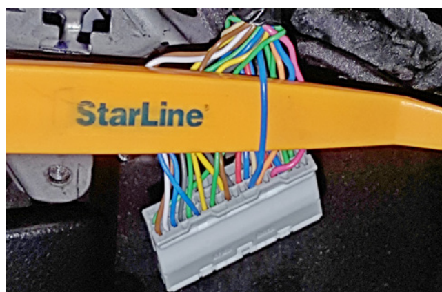
Фото 3.10. Зажигание 2 (синий)
