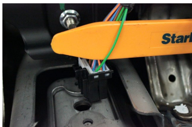
Фото 3.5. Контроль концевика багажника (зелёный)
