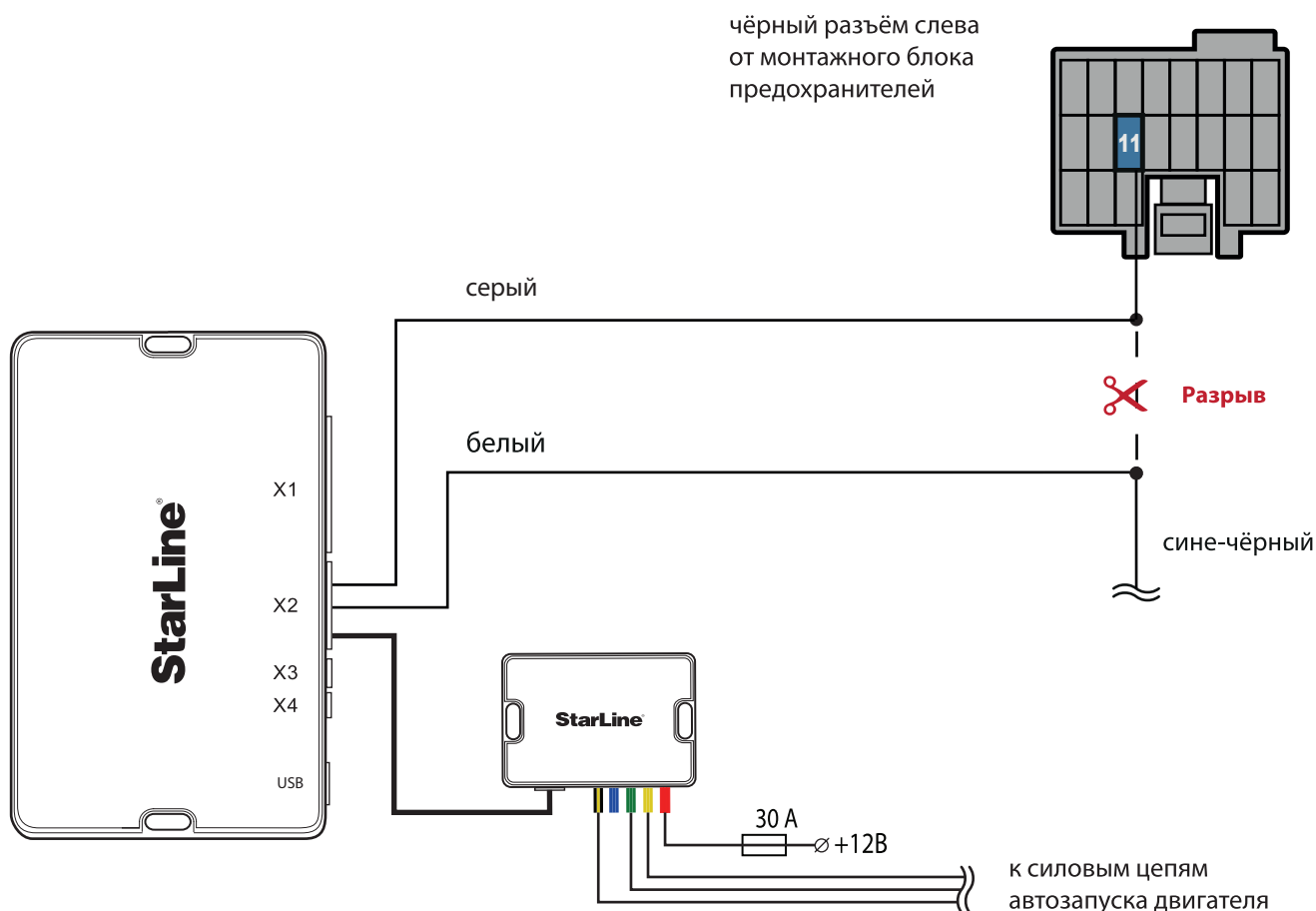
Схема 1. Подключение цепей автозапуска двигателя и обхода штатного иммобилайзера
