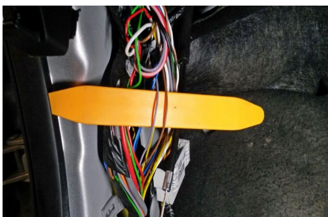
Фото 3.9. Управление центральным замком (серый и коричневый)
