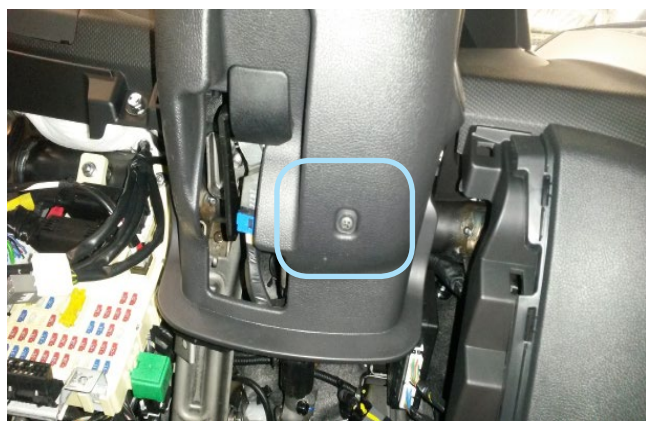
Фото 1.11. Саморез крепления нижней части кожуха рулевого вала снизу
