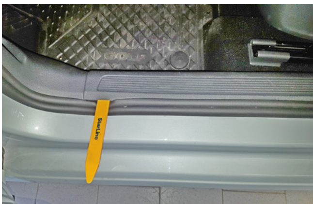
Фото 1.7. Снять накладку порога двери водителя
