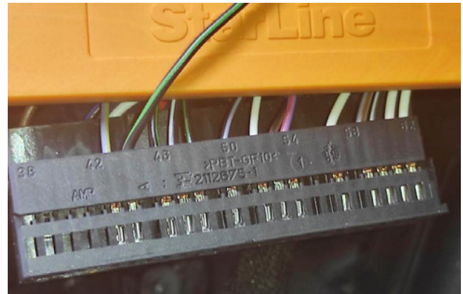
Фото 3.9. Зажигание 1 (чёрно-зелёный)
