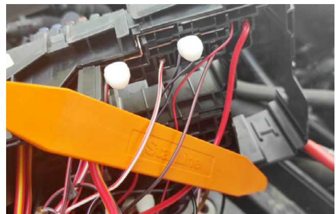
Фото 3.13. Цепи управления стартером (бело-красный и чёрно-красный)
