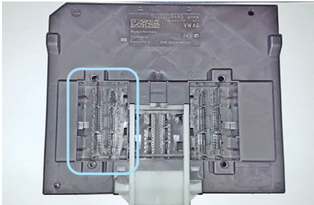
Фото 3.2. Местоположение разъёма А на блоке ВСМ
