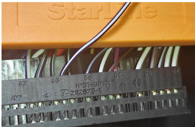
Фото 3.10. Зажигание 2 (чёрно-белый)
