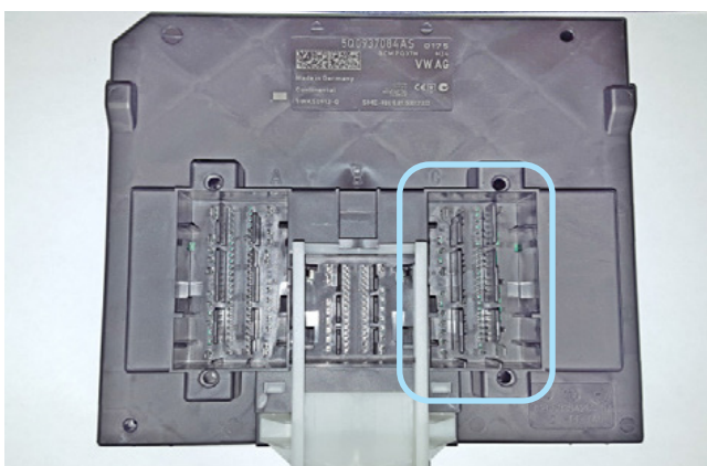
Фото 3.6. Местоположение разъёма С на блоке ВСМ
