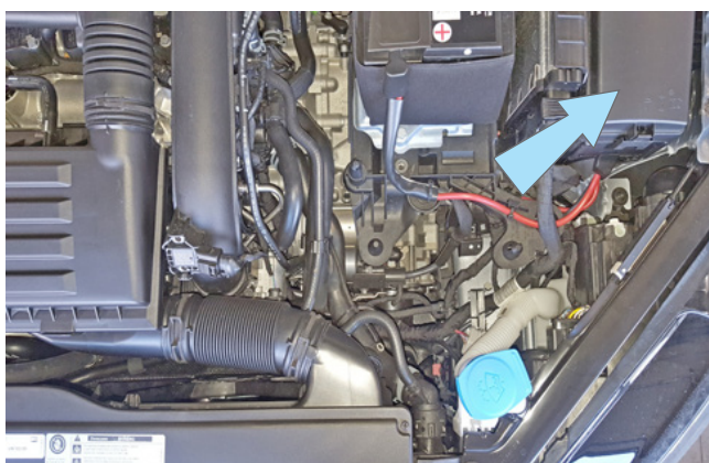
Фото 3.12. Местоположение монтажного блока предохранителей под капотом
