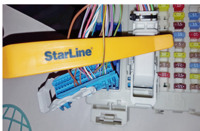
Фото 3.5. Управление световыми сигналами (коричнево-жёлтый)
