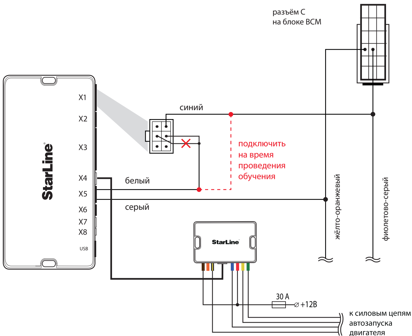
Фото 3.6. Шина данных штатного иммобилайзера (фиолетово-серый и жёлто-оранжевый)
