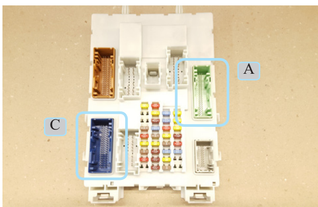
Фото 3.2. Местоположение разъёмов на блоке ВСМ
