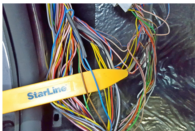
Фото 3.7. Управление световыми сигналами (коричневый и синий)
