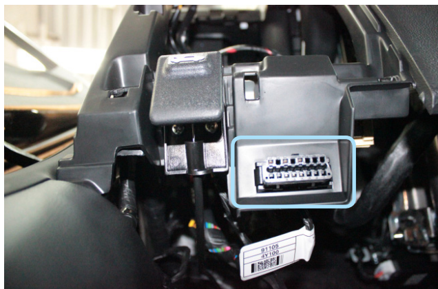
Фото 3.4. Местоположение диагностического разъёма
