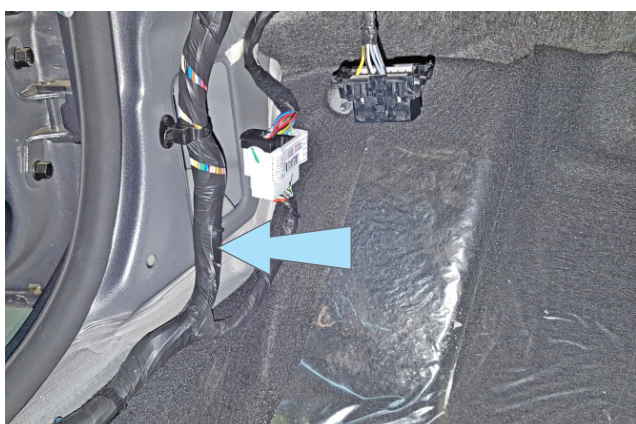
Фото 3.6. Местоположение жгута в левой кик-панели
