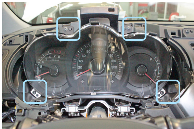
Фото 1.19. Саморезы крепления панели приборов
