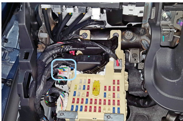
Фото 3.8. Местоположение разъёма
