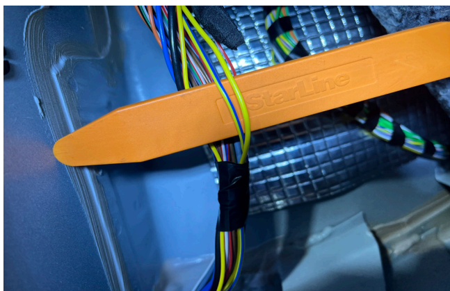
Фото 3.4. Провода управления ЦЗ (жёлтый и жёлто-синий)
