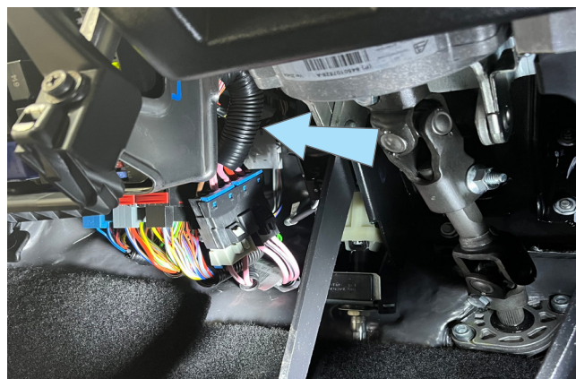
Фото 3.11. Местоположение блока комфорта
