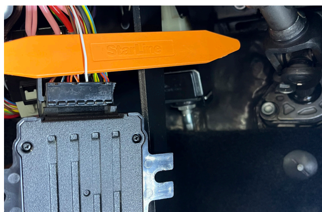
Фото 3.13. ЦЗ открытие (белый pin-5)
