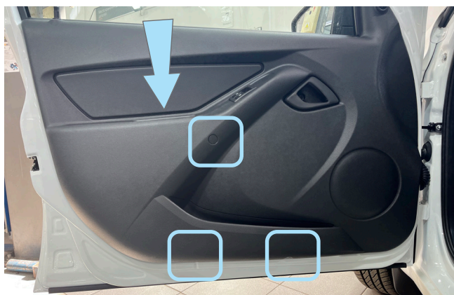
Фото 3.8. Саморезы крепления обшивки двери водителя
