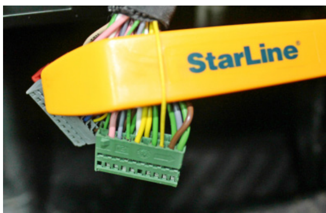
Фото 3.10. Контроль концевика передней правой двери (жёлтый)
