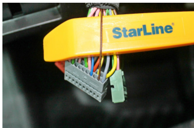
Фото 3.9. Контроль концевика передней левой двери (коричневый)
