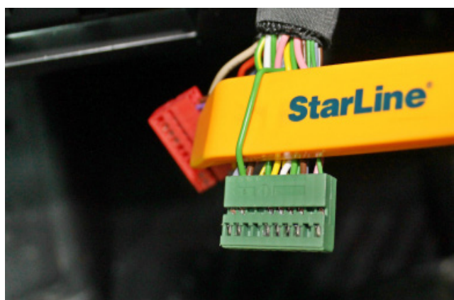
Фото 3.11. Контроль концевика багажника (зелёный)
