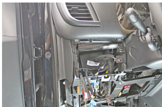
Фото 1.6. Блок кнопок снят
