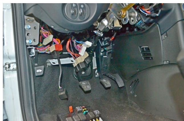
Фото 1.18. Монтажный блок снят
