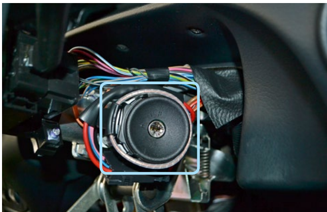
Фото 3.16. Расположение антенны модуля VP-03 на замке зажигания
