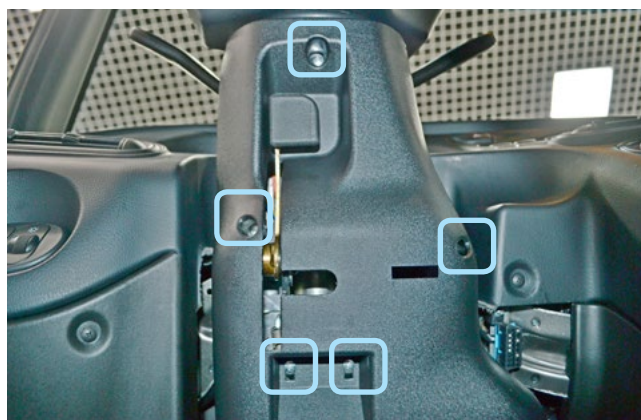
Фото 1.4. Крепление нижней части рулевого кожуха
