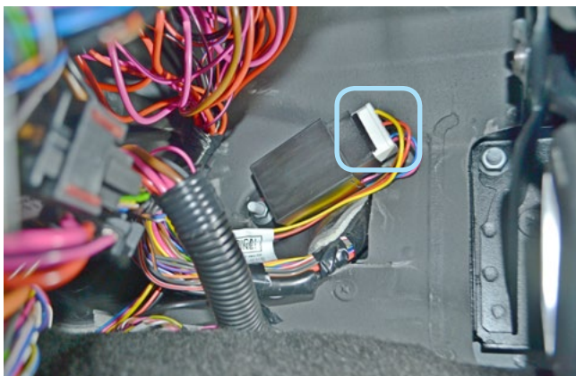
Фото 3.10. Блок управления центральным замком
