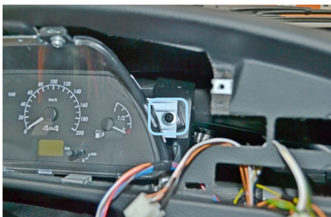
Фото 1.13. Саморез крепления панели приборов справа
