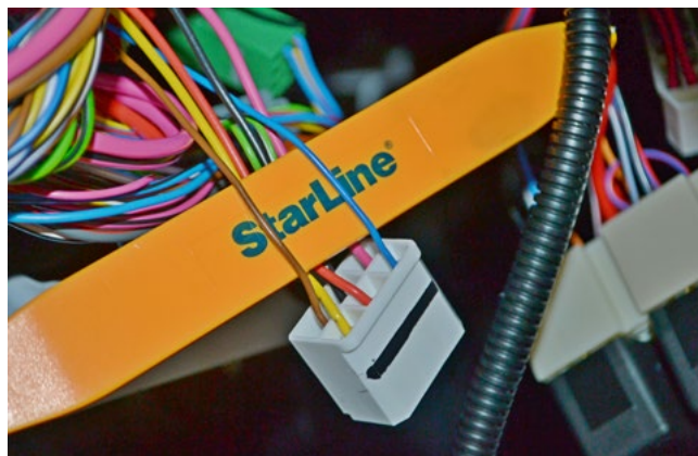
Фото 3.11. Управление центральным замком (коричневый и синий)
