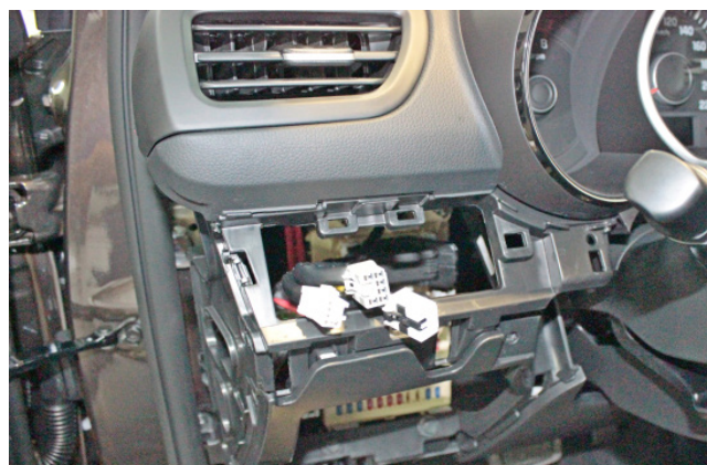
Фото 1.7. Блок кнопок управления снят
