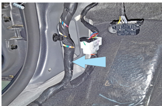
Фото 3.5. Местоположение жгута в левой кик-панели
