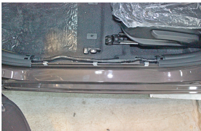
Фото 1.12. Накладка порога двери водителя снята
