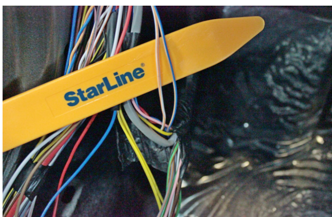
Фото 3.7. Управление центральным замком (бело-оранжевый и сине-оранжевый)
