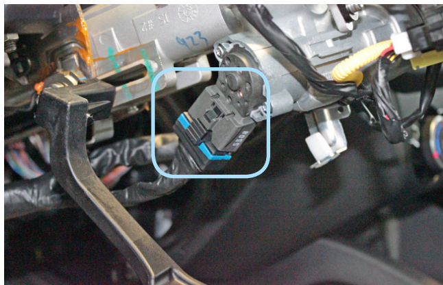
Фото 3.13. Местоположение разъёма
