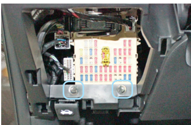
Фото 1.8. Болты крепления пластиковой накладке под рулевой колонкой
