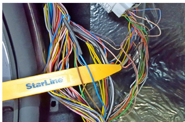
Фото 3.6. Управление световыми сигналами (коричневый и синий)
