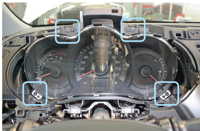
Фото 1.25. Саморезы крепления панели приборов
