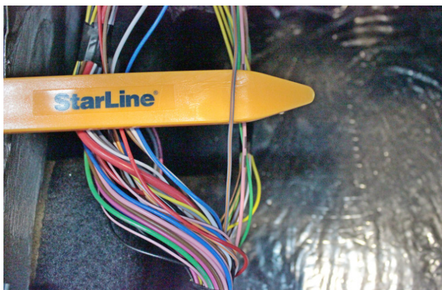
Фото 3.8. Контроль стояночного тормоза (серо-оранжевый)
