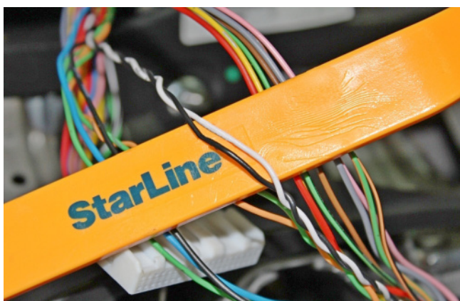
Фото 3.4. Шина CAN-B (белый и чёрный)
