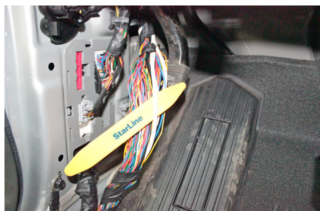
Фото 3.14. Питание +12В (белый)
