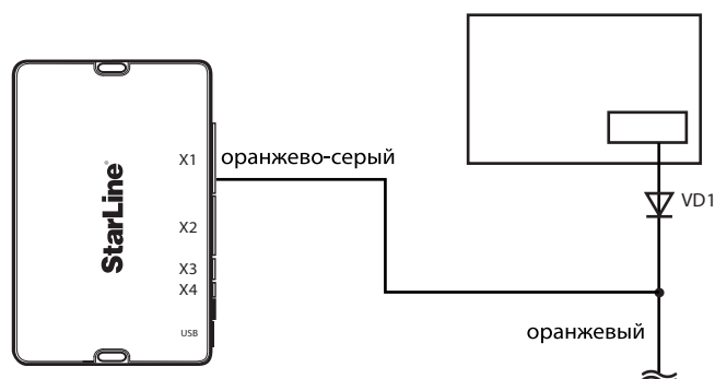
Схема 2. Подключение к концевика капота (оранжевый)
