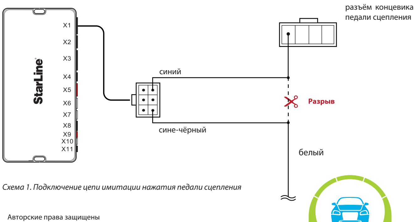
Фото 3.8. Имитация нажатия педали сцепления (белый)
