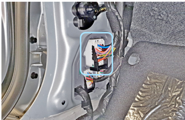
Фото 3.5. Местоположение разъёма
