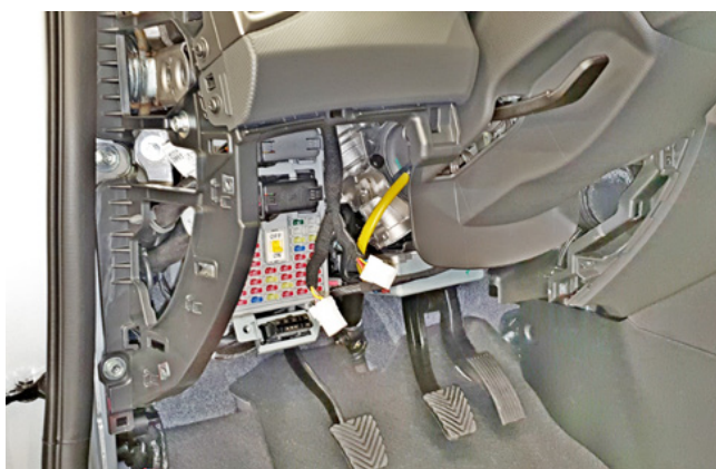
Фото 1.11. Пластиковая накладка под рулевой колонкой снята
