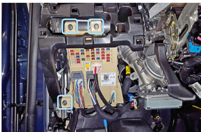
Фото 1.28. Крепление монтажного блока предохранителей
