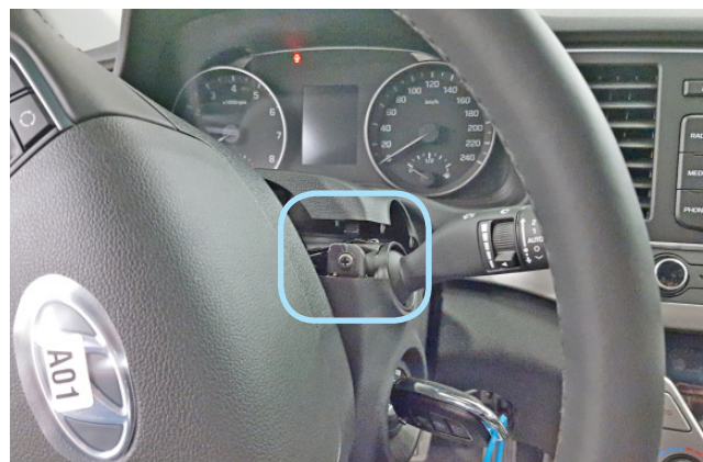
Фото 1.14. Саморез крепления нижней части кожану рулевого вала справа
