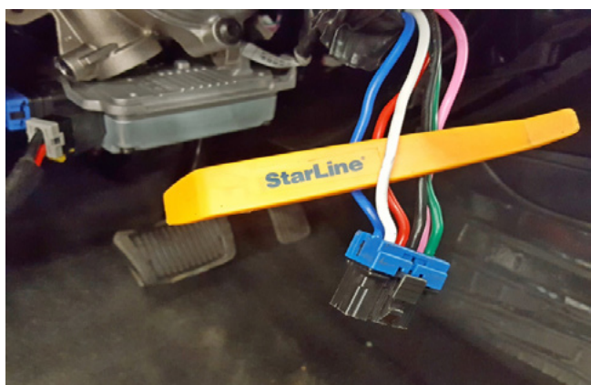
Фото 3.12. Стартер (белый)
