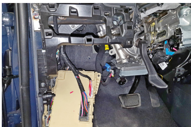
Фото 1.29. Монтажный блок предохранителей снят
