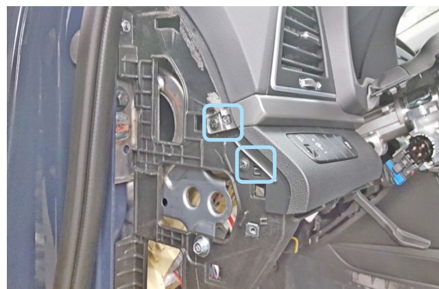
Фото 1.18. Саморезы крепления декоративной накладки и блока кнопок управления
