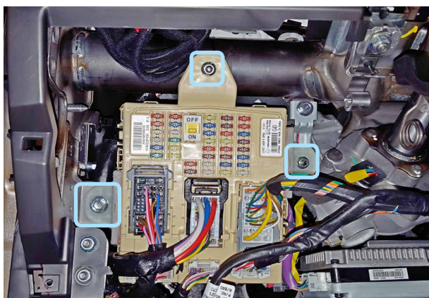
Фото 2. Крепление монтажного блока предохранителей
