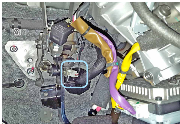
Фото 11.1. Местоположение разъёма
