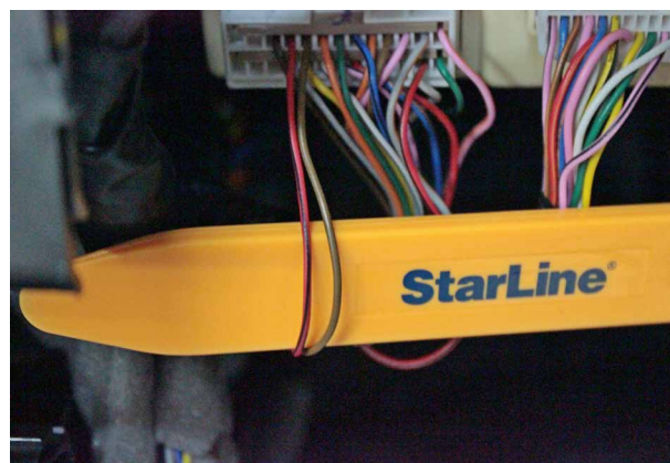
Фото 9.2. Управление центральным замком (красно-чёрный и коричнево-чёрный)
