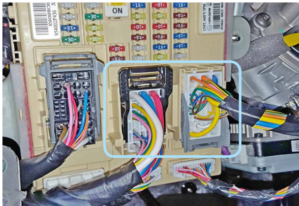
Фото 13.1. Местоположение разъёмов
