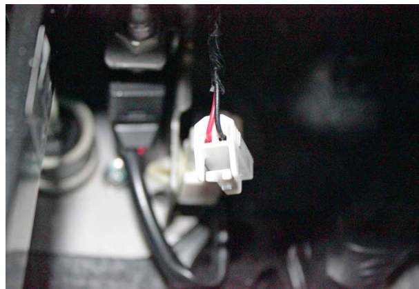
Фото 11.2. Имитация нажатия педали сцепления (красный и чёрный)
