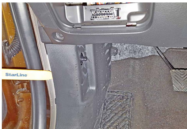
Фото 1.5. Снять накладку левой кик-панели
