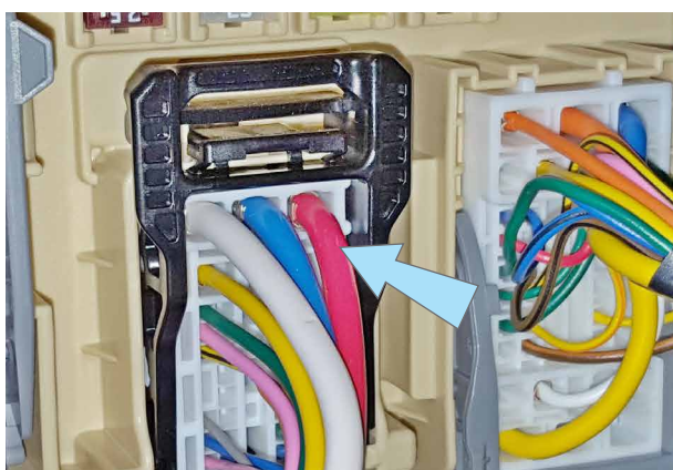
Фото 13.5. Питание +12В (красный)
