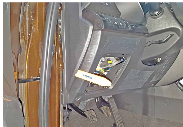
Фото 1.6. Снять боковую накладку передней панели
