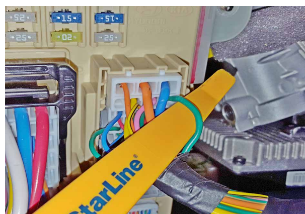
Фото 13.4. Стартер (зелёный)
