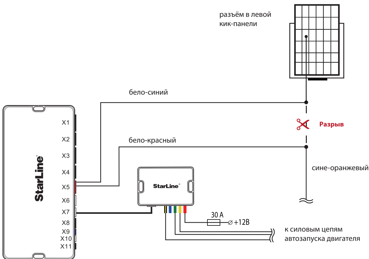
Схема 2. Подключение цепей автозапуска двигателя и обхода штатного иммобилайзера
