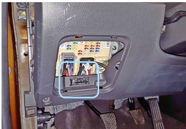
Фото 7.1. Местоположение диагностического разъёма
