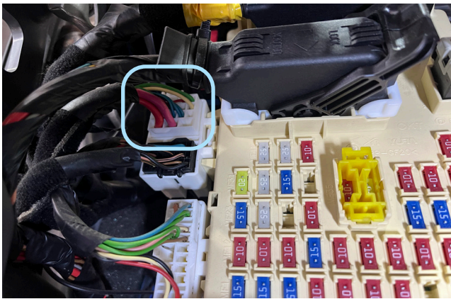
Фото 3.12. Местоположение разъёма
