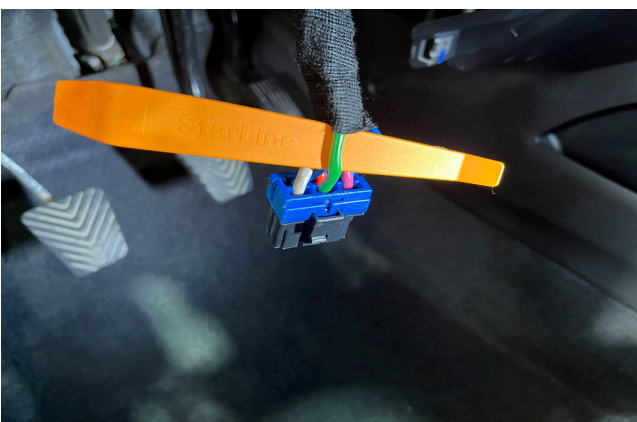
Фото 3.16. Зажигание 2 (зелёный)
