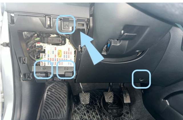
Фото 1.5. Крепления накладки под рулевой колонкой
