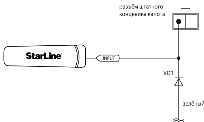
Схема 1. Подключение к штатному концевика капота
