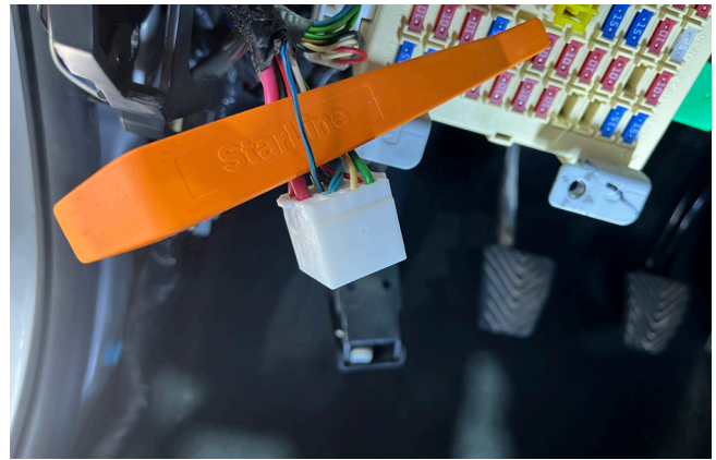
Фото 3.13. Шина LIN (сине-чёрный)
