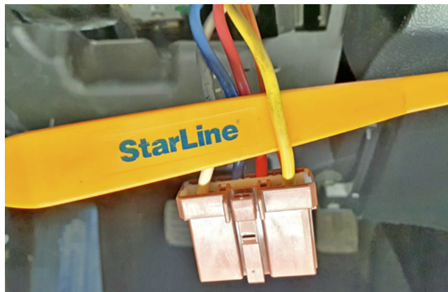
Фото 3.12. Стартер (жёлтый)
