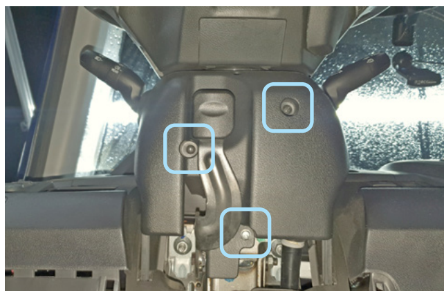
Фото 1.9. Саморезы крепления нижней части кожуа снизу
