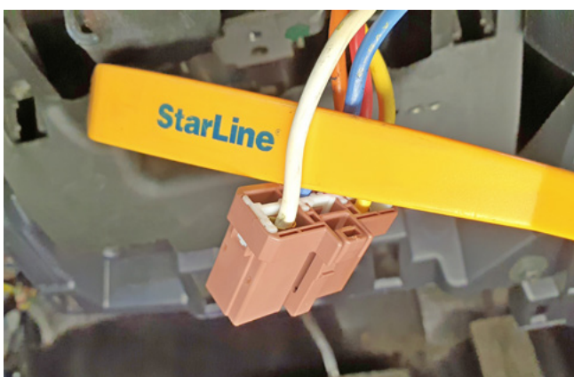
Фото 3.13. Питание +12В (белый)
