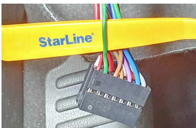
Фото 3.11. Питание +12В (зелёный)
