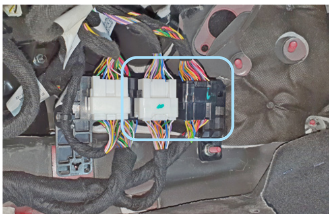
Фото 3.7. Местоположение разъемов
