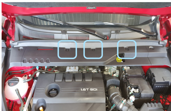
Фото 2.2. Клипсы крепления пластиковой накладки
