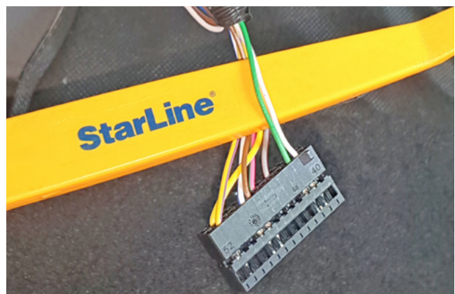
Фото 3.4. Шина CAN-A (зелёный и белый)
