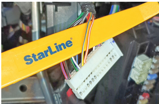
Фото 3.10. Провода антенны штатного иммобилайзера (жёлто-синий и оранжево-белый)
