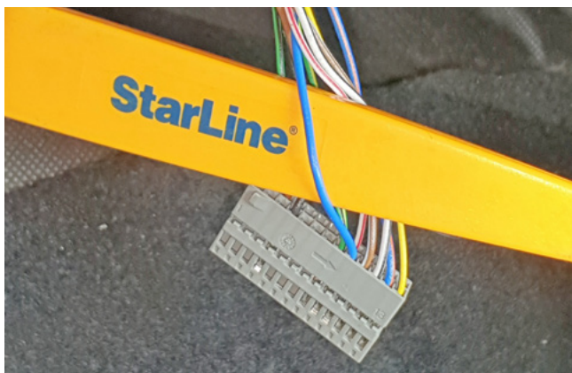
Фото 3.5. Альтернативное управление световыми сигналами (синий)
