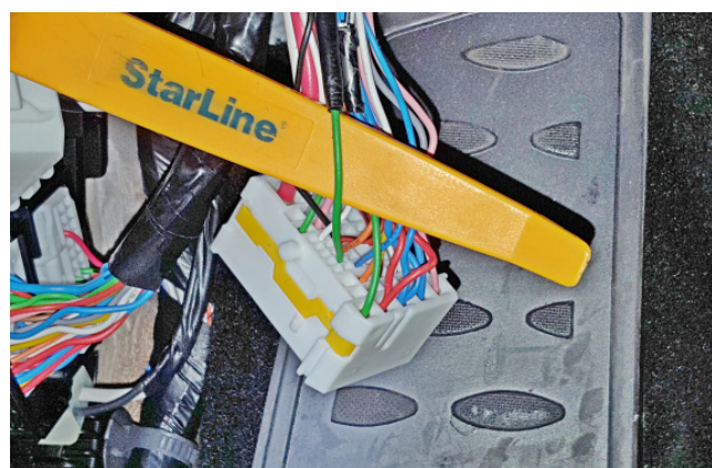
Фото 3.9. Контроль педали тормоза (зелёный)
