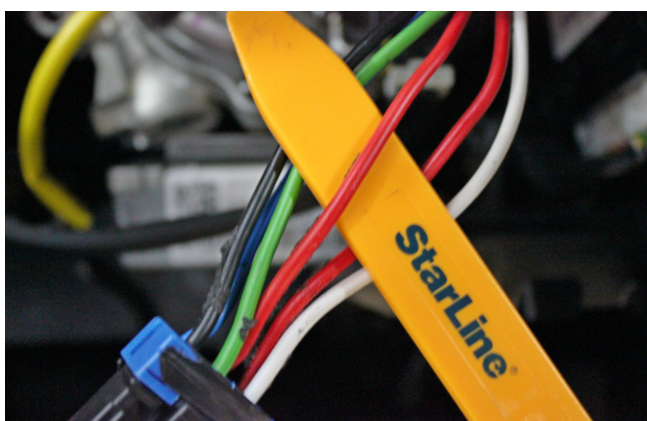
Фото 3.16. Питание +12В (красный)
