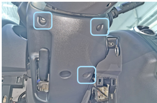
Фото 1.8. Саморезы крепления нижней части кожуха рулевого вала
