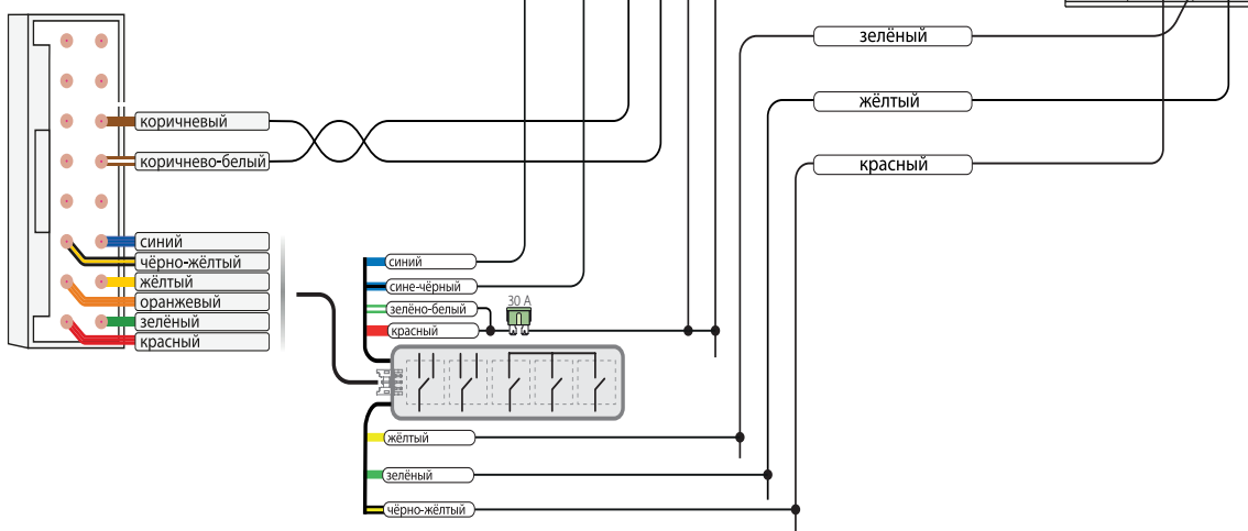
Схема 1. Подключение цепей автозапуска двигателя
