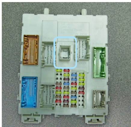
Фото 3.11. Местоположение разъёма на блоке VCM
