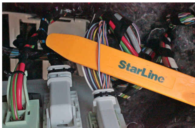
Фото 3.9. Имитация нажатия педали тормоза (фиолетово-белый)
