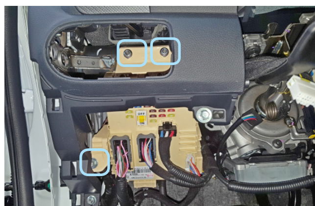
Фото 1.12. Блок кнопок снят. Крепление монтажного блока предохранителей
