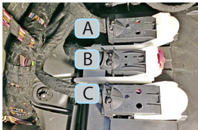
Фото 3.3. Наименование разъёмов на блоке BCM
