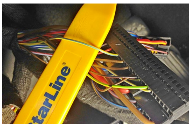
Фото 3.8. Разъём А, аксессуары (жёлто-синий)
