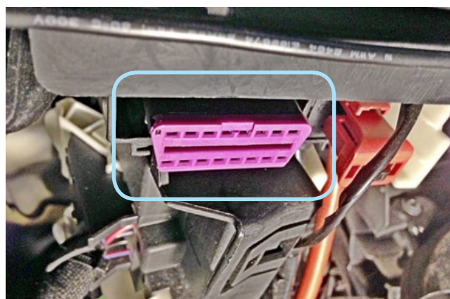
Фото 3.5. Местоположение диагностического разъёма
