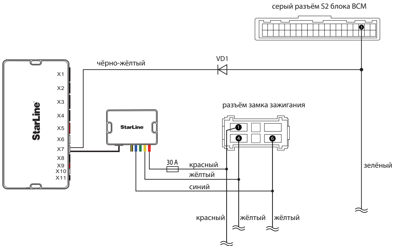
Схема 1. Подключение цепей автозапуска двигателя
