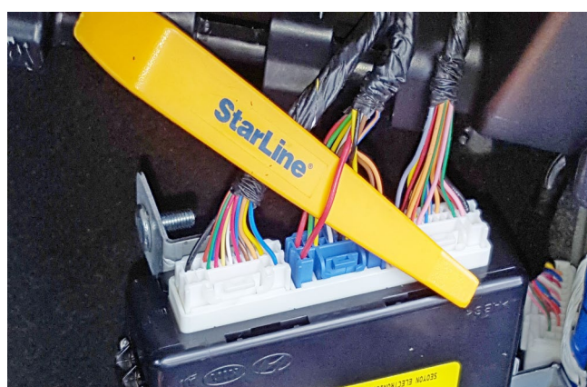
Фото 3.10. Питание +12В (красный)
