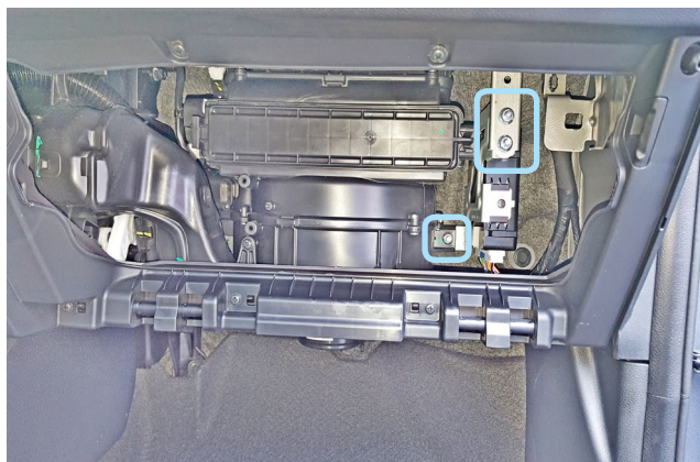
Фото 1.2. Крепление блока SmartKey
