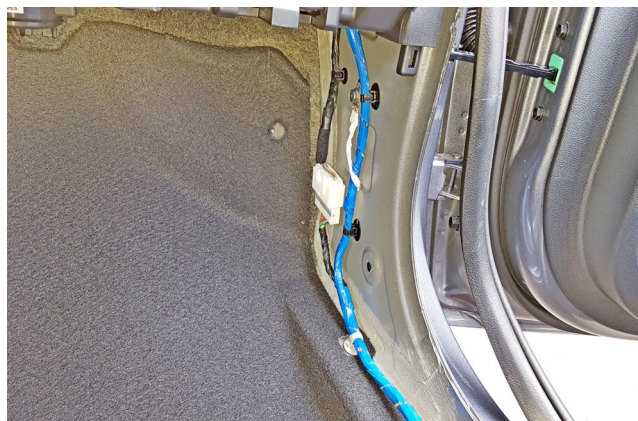
Фото 1.8. Накладка правой кик-панели снята
