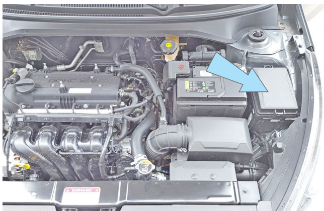
Фото 2.5. Возможное место установки подкапотного блока R6
