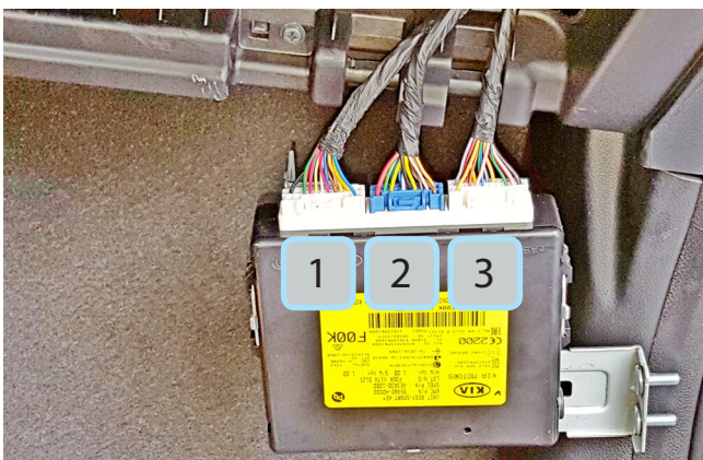
Фото 3.2. Условная нумерация разъемов блока SmartKey
