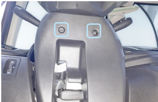
Фото 1.1. Саморезы крепления нижней части кожуха
