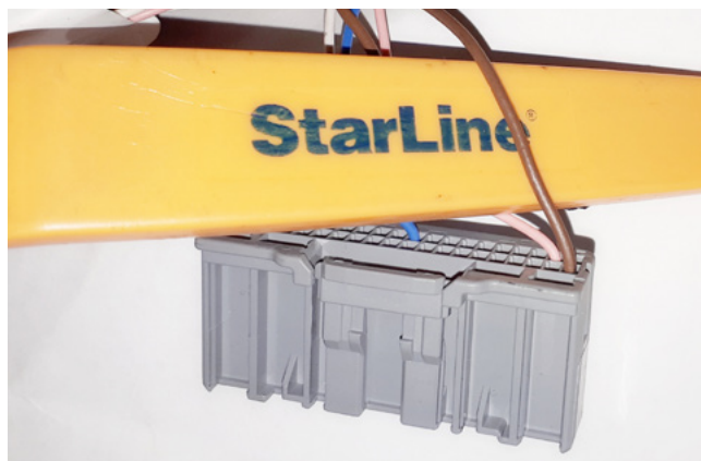
Фото 3.6. Концевик капота (коричневый)
