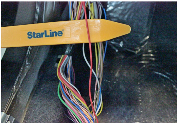
Фото 12. Контроль педали тормоза (красный)
