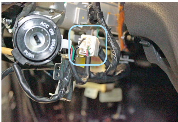
Фото 15.1. Местоположение разъёма
