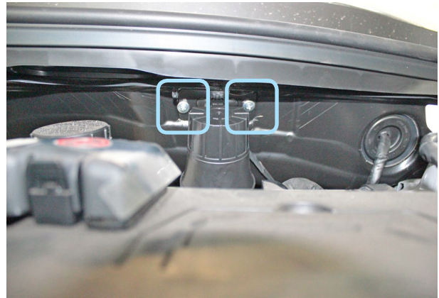
Фото 5.2. Крепление сирены
