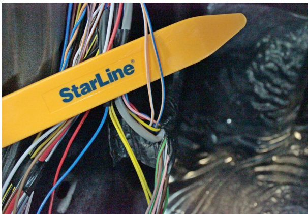
Фото 11. Управление центральным замком (бело-оранжевый и сине-оранжевый)
