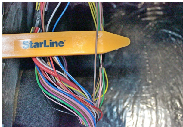
Фото 13. Контроль стояночного тормоза (серо-оранжевый)
