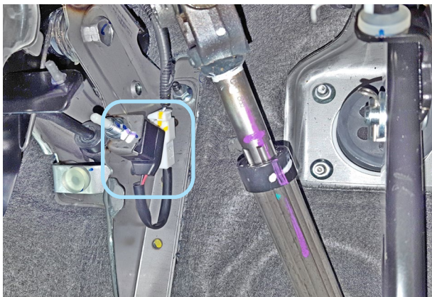
Фото 14.1. Местоположение разъёма концевика педали сцепления
