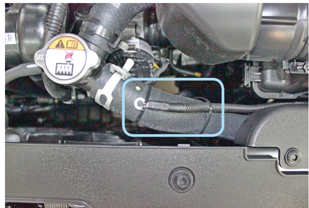
Фото 5.4. Крепление датчика температуры двигателя
