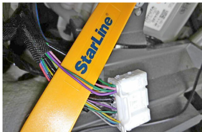
Фото 3.5. Шина LIN (фиолетовый и зелёный)
