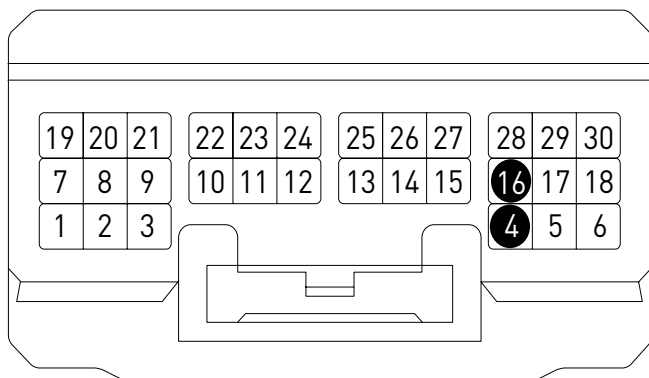
Рисунок 1. Pin 4 - Rx (белый), pin 16 - Tx (бело-зелёный)
