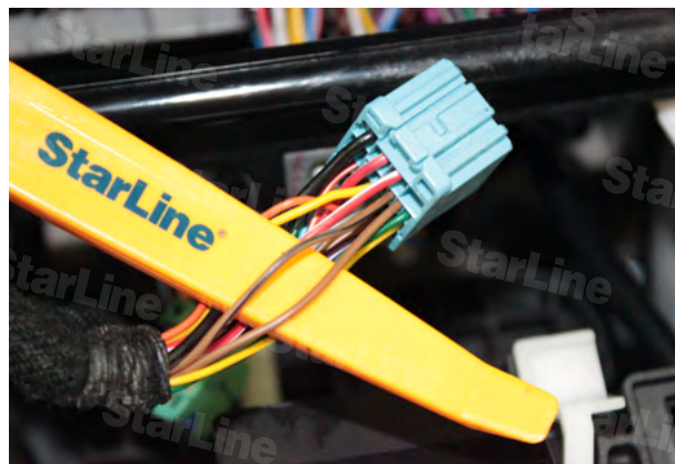
Фото 9.2. Шина CAN-B (коричнево-чёрный и коричневый)
