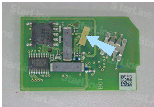
Фото 15.2. Контактная площадка (+) на плате ключа
