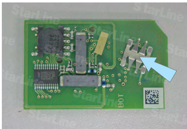
Фото 15.1. Контактная площадка (-) на плате ключа
