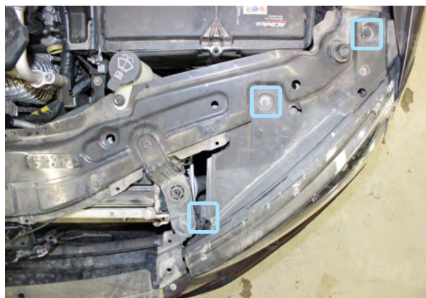
Фото 5.2. Болты крепления блок-фары
