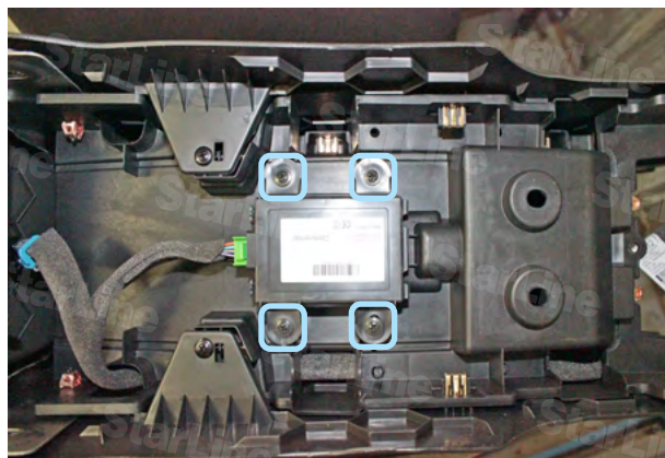
Фото 14.1. Крепление блока штатного иммобилайзера
