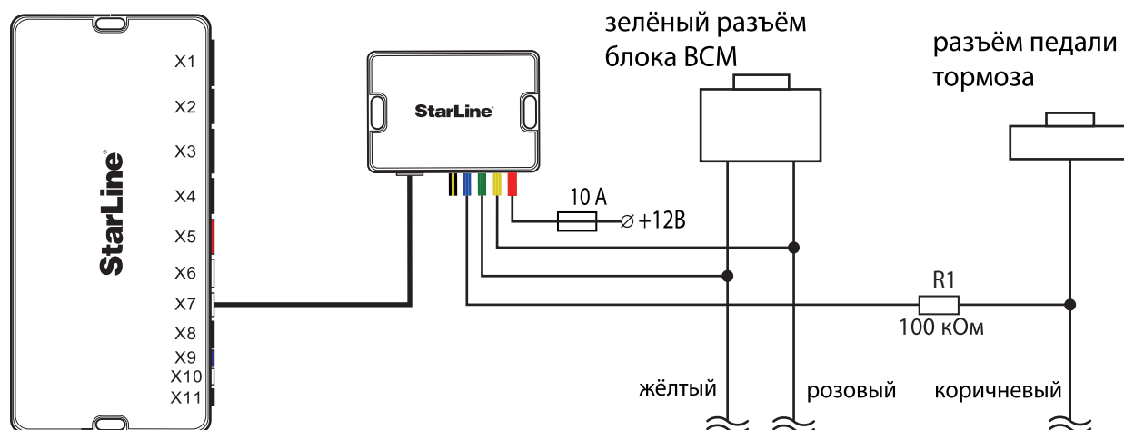
Схема 1. Цепи автозапуска двигателя
