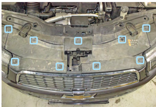
Фото 5.1. Клипсы крепления декоративной накладки радиатора
