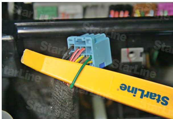
Фото 9.1. Шина CAN-A (зелёный)
