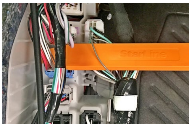
Фото 3.7. Управление центральным замком - отпирание (серый)
