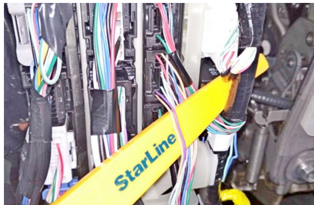
Фото 3.3. Шина CAN-A (бежевый и фиолетовый)
