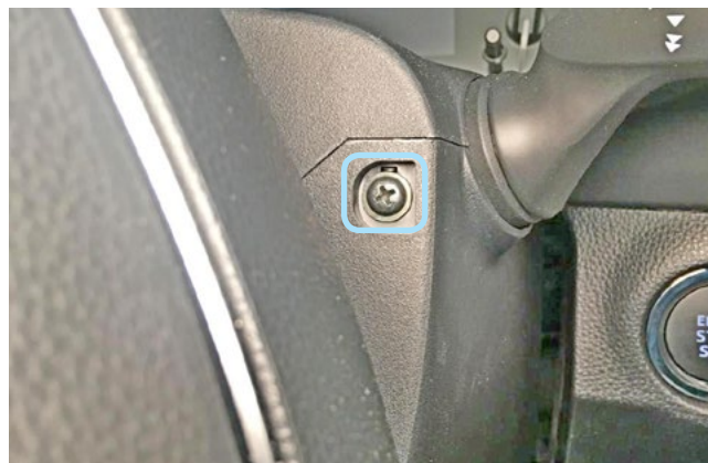
Фото 1.18. Саморез крепления кожуха рулевого вала справа
