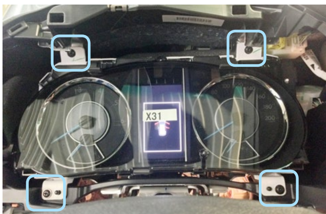
Фото 1.16. Накладка панели приборов снята. Саморезы крепления
