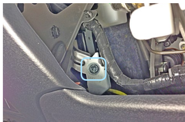
Фото 1.9. Болт крепления подушки безопасности сверху слева
