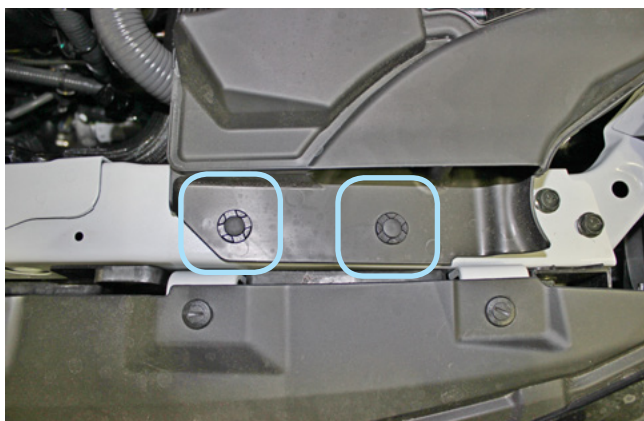
Фото 2.3. Клипсы крепления воздуховода
