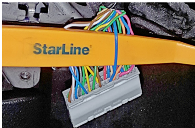
Фото 3.10. Зажигание 2 (синий)
