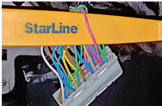
Фото 3.8. Аксессуары (розовый)
