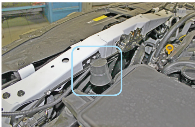
Фото 2.5. Возможное место установки сирены
