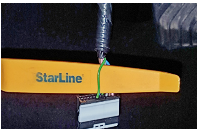
Фото 3.11. Стартер (зелёный)
