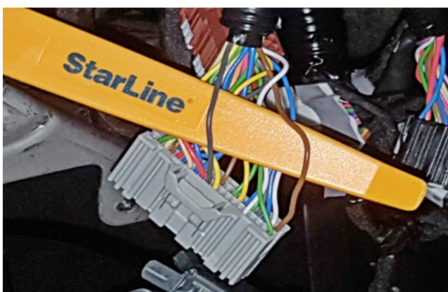
Фото 3.6. Управление центральным замком (серый и коричневый)
