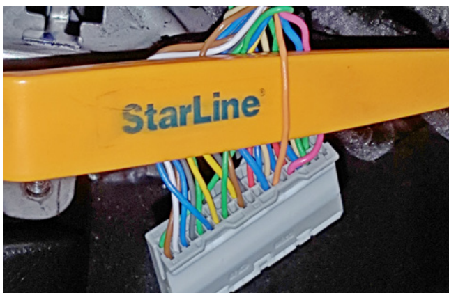
Фото 3.9. Зажигание 1 (оранжевый)
